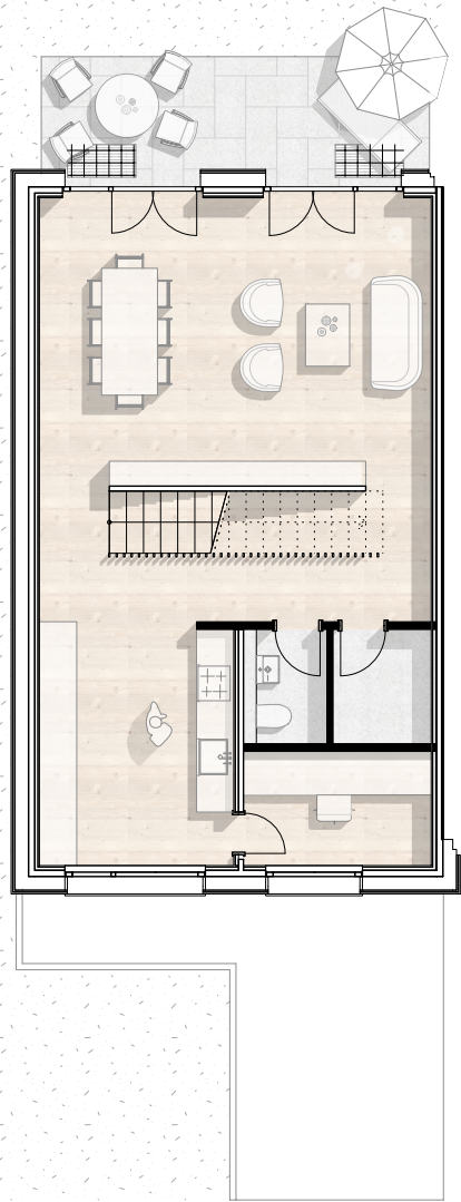
Wohngeschoss Standard
